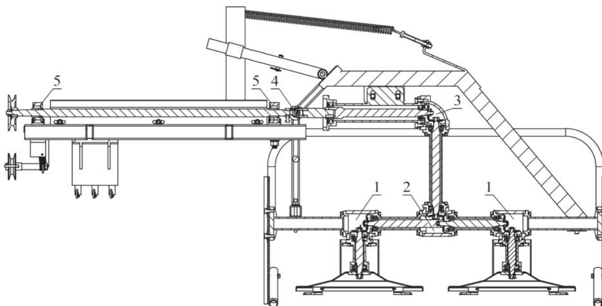
Рисунок 2. Места смазки задней роторной косилки
