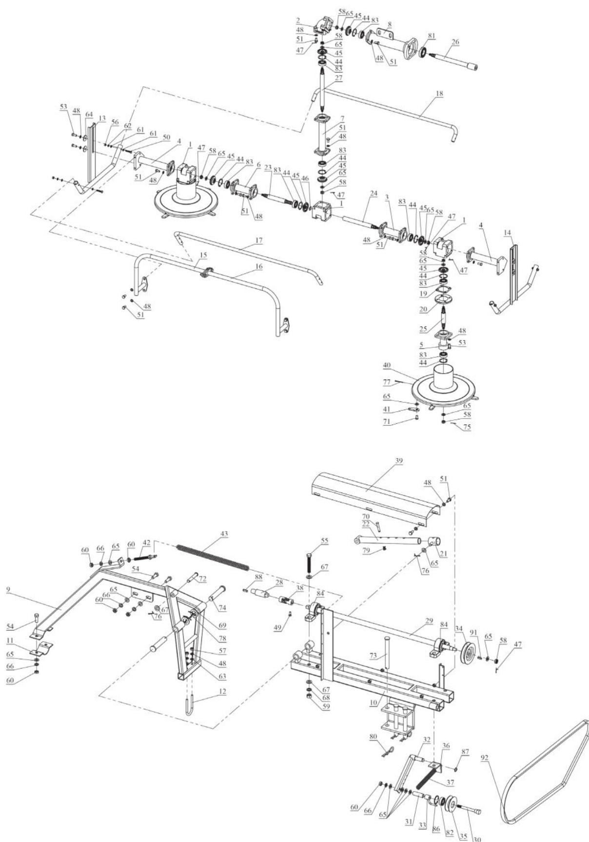
Рисунок 3. Комплектующие задней роторной косилки к мини-тракторам РУСИЧ
